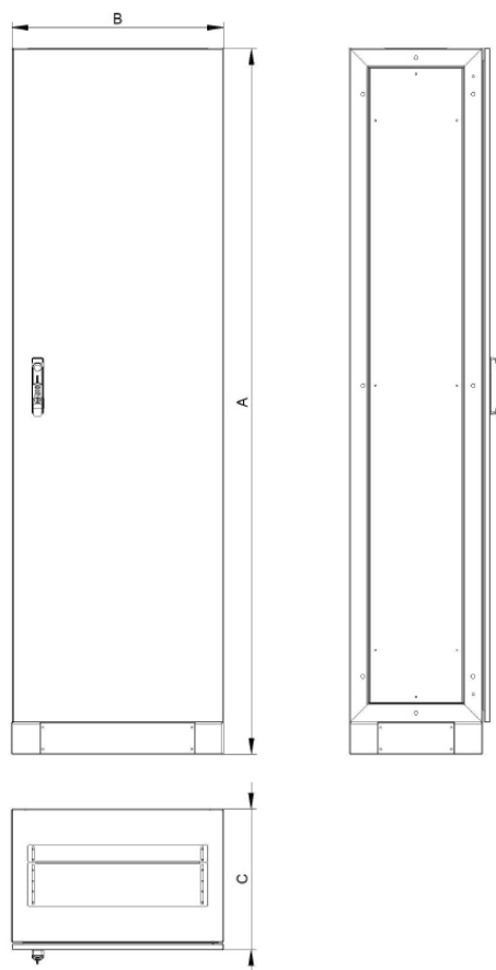
Wymiary
